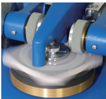
テーパー摩耗試験機 ■試験条件 テーパー CS-17 1kg×1,000回
